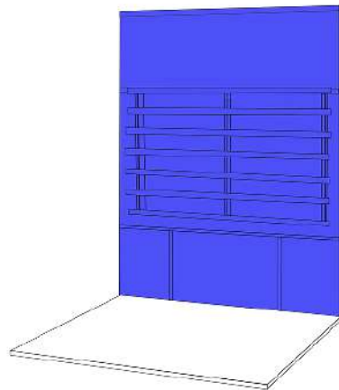
(2) Ustaw ścianę tylną na panelu podłogowym
