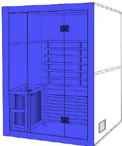
(9) Umieść przedni panel na panelu podłogowym i połącz go za pomocą klamr
