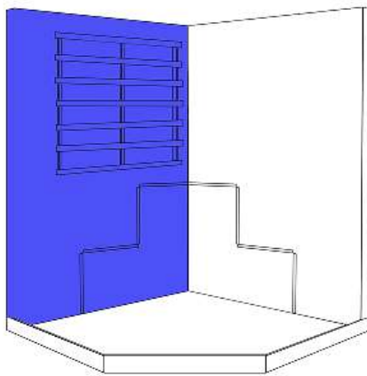
(3) Ustaw lewą tylną ścianę na panelu podłogowym i połącz ściany klamrami
