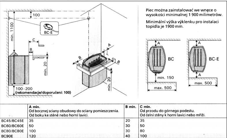
Rys. 6. Minimalne odległości instalacyjne (wymiar w milimetrach)
