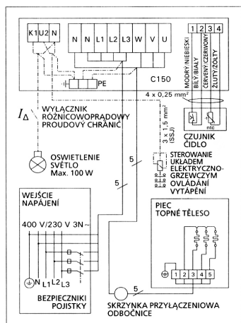
Rys. 10. Schemat elektryczny (BC) Obrázek 10. Zapojení topného tělesa BC
