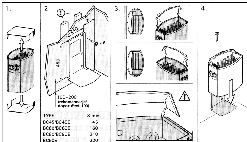
Rys. 7. Mocowanie pieca na ścianie (wymiary w milimetrach)
