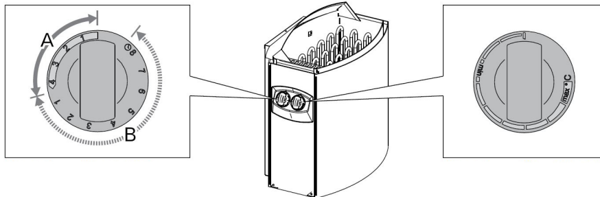
Rys. 2. Przełącznik zegara
