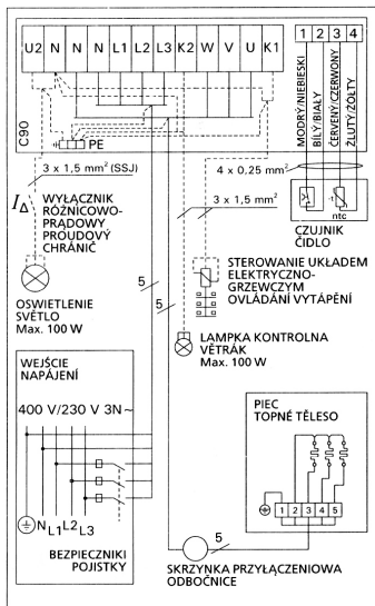
Rys. 12b. Schemat elektryczny pieca typu BC-E i modulu sterującego C90
