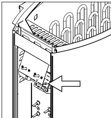
Rys. 9. Przycisk resetowania wyłącznika termicznego
