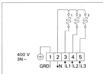
Rys. 11. Schemat elektryczny (BC-E) Obrázek 11. Zapojení topného tělesa BC-E
