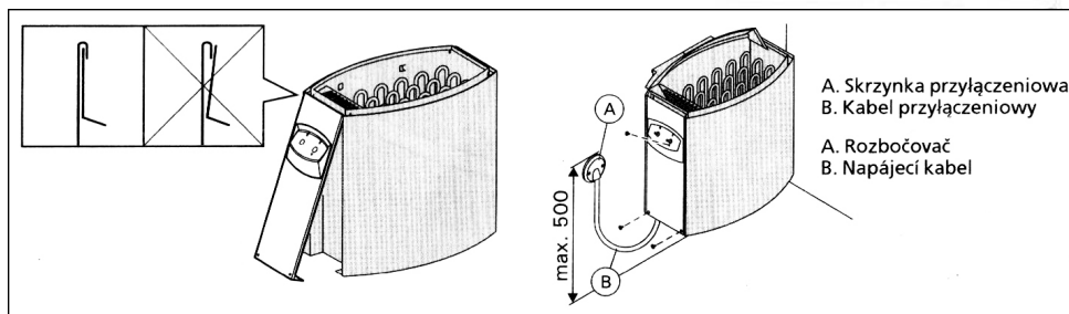
Rys. 8. Zamykanie pokrywy skrzynki przyłączeniowej (wymiary w milimetrach)
